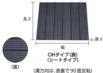
OHSタイプ(表) (ミニシートタイプ) (溝方向は、表裏で90度反転)
