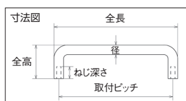
B-1796 (鏡面仕上げ)
