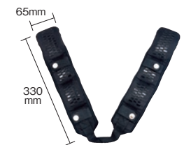
KPCR-F
